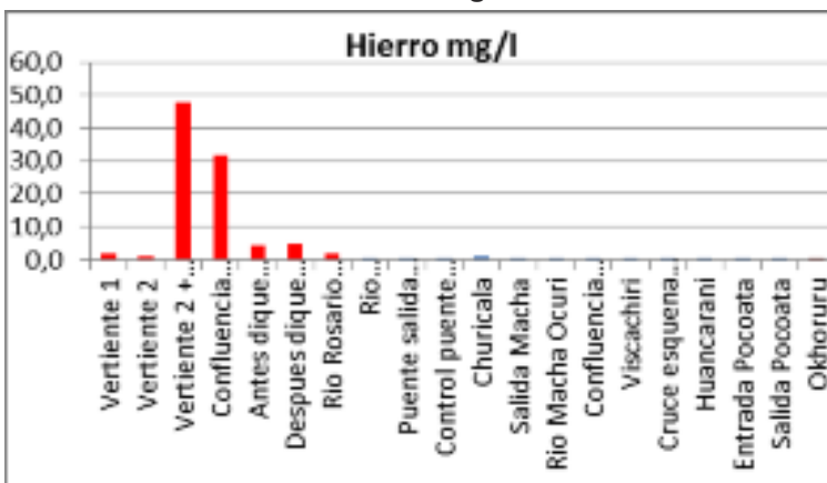
Gráfico N° 6. Agua: Hierro
