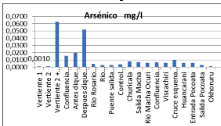
Gráfico N° 4. Agua: Arsénico
