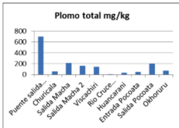
Gráfico N° 13. Suelos: Plomo
