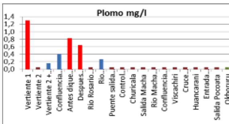
Gráfico N° 7. Agua: Plomo
