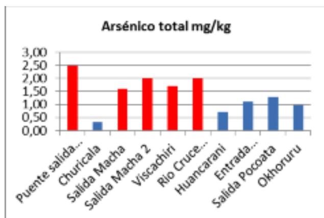
Gráfico N° 15. Plantas: Arsénico
