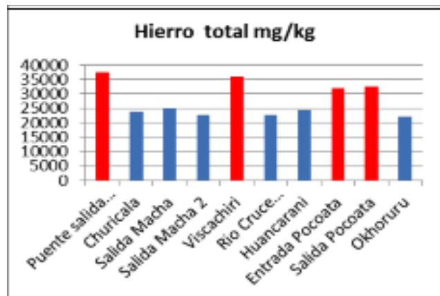
Gráfico N° 11. Suelos: Hierro
