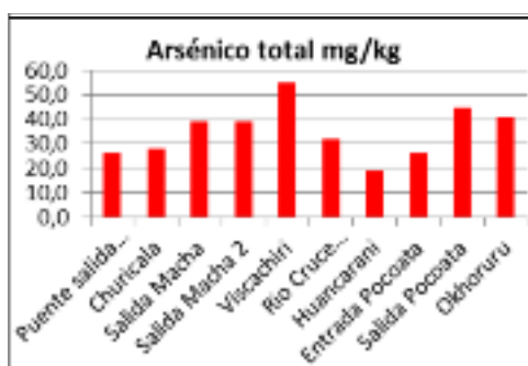
Gráfico N° 9. Suelos: Arsénico
