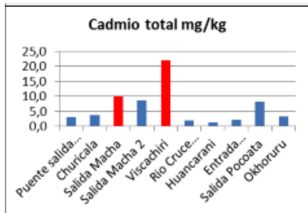
Gráfico N° 10. Suelos: Cadmio
