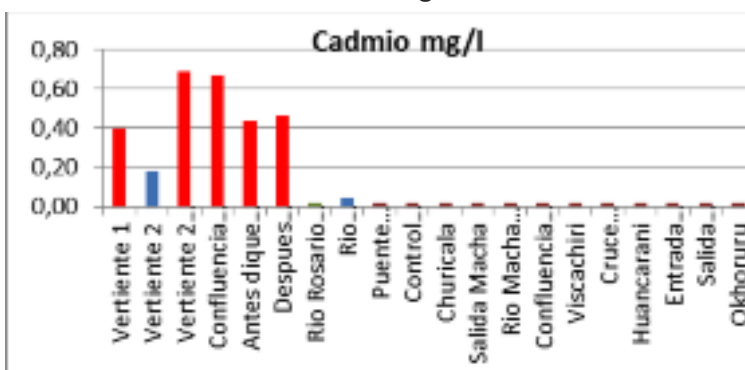
Gráfico N° 5. Agua: Cadmio
