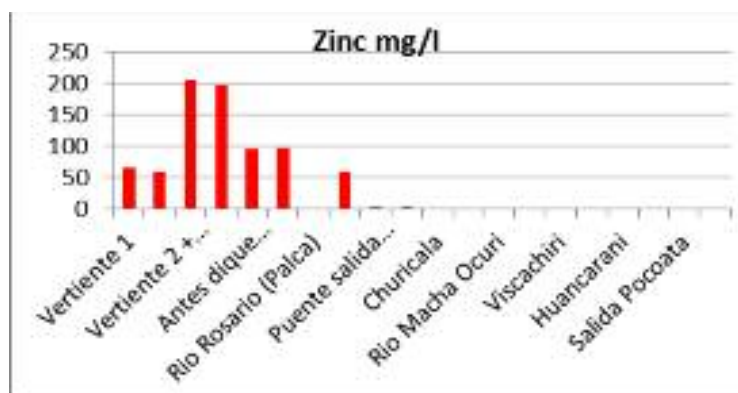
Gráfico N° 8. Agua: Zinc
