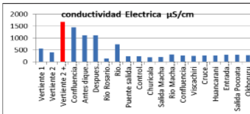
Gráfico N° 2. Agua: Conductividad
