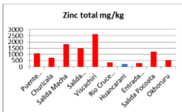
Gráfico N° 14. Suelos: Zinc
