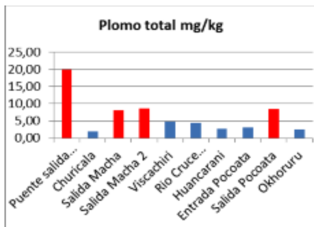
Gráfico N° 17. Plantas: Plomo
