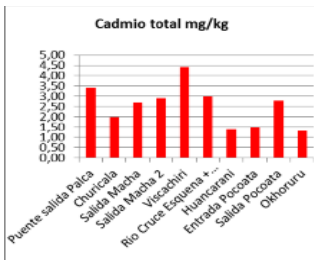
Gráfico N° 16. Plantas: Cadmio
