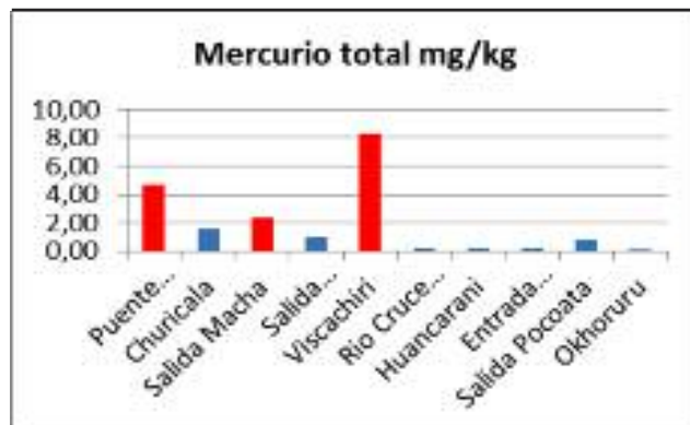
Gráfico N° 12. Suelos: Mercurio
