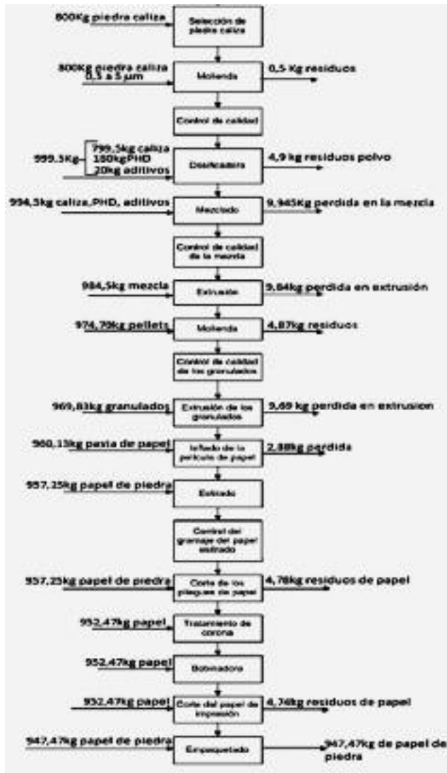
Gráfico N° 2. Diagrama de flujo del Balance Másico
