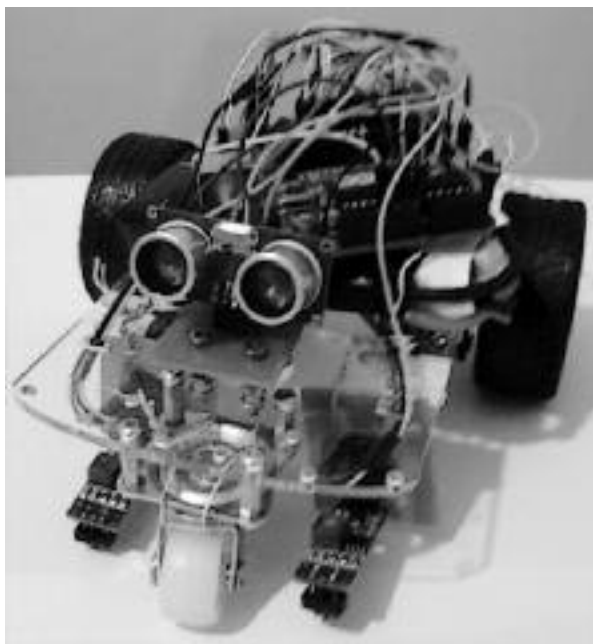
Figura N° 4. Diseño Final
