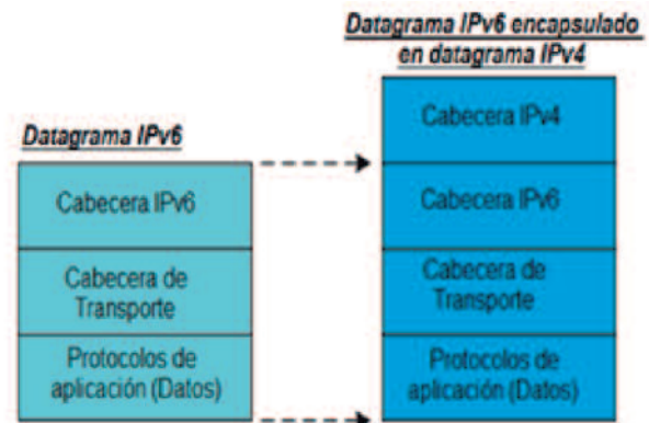
Figura N°1. Encapsulamiento del datagrama IPv6
