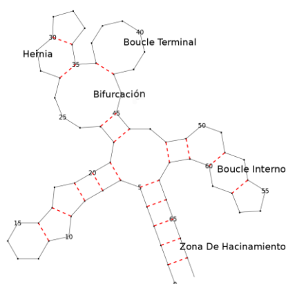
Figura 2: Esquema de una estructura secundaria de ARN, mostrando las cinco clases de "figuras" existentes. Este esquema fue realizado por el algoritmo de representación gráfica de estructuras secundarias de ARN.
