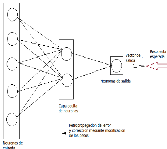
Figura 4: Esquema de la red multicapa unidireccional utilizada.
