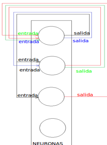
Figura 3. Esquema de la red de Hopfield utilizada. Cada neurona envía un vector de salida a las neuronas con las cuales sufre una contradicción.
