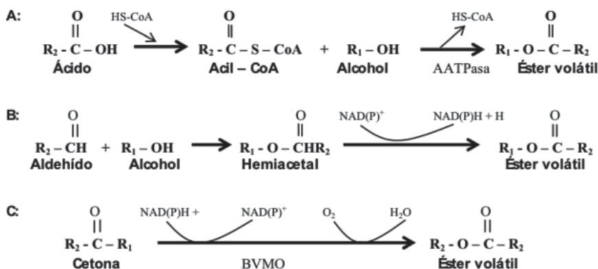
Figura 1. Mecanismos de producción de ésteres de carboxilato por tres rutas metabólicas, a. Alcohol Acetiltransferasa (AATasa), b. Alcohol deshidrogenasa (ADH), y c. Baeyer – Villiger Monooxigenasa (Park, et al, 2009).
