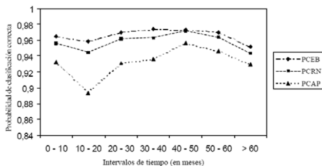
Figura 2. Probabilidad de clasificación correcta estimadas para los diferentes intervalos de tiempo según que hayamos utilizado la regla de Bayes (PCEB), la regla de Bayes obtenida por la red neuronal (PCRN) y las probabilidades a priori (PCAP).
