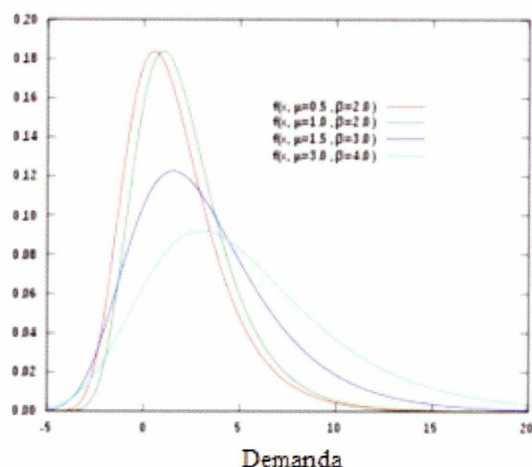
Figura 3. Distribución de Gumbel
