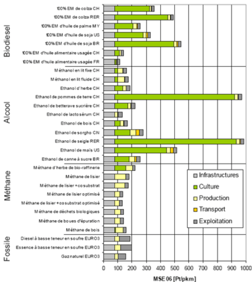
Illustration 3. Comparaison de la charge environnementale agrégée (méthode de la saturation écologique (MSE 06)) des biocarburants et des carburants fossiles (essence et diesel, EURO 3), ventilée selon les différents processus qui interviennent le long de la chaîne de production.
